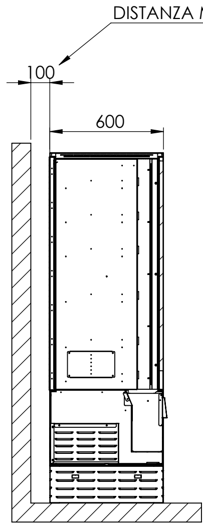
SEZIONE A-A
